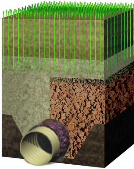
(fotoğraf: Desso GrassMaster uygulama kesiti)
